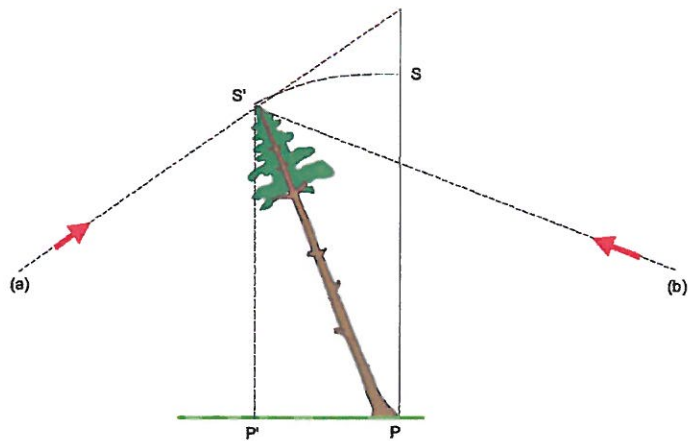
4. ábra A magasságmérés hibája a fa dőléséből eredően
