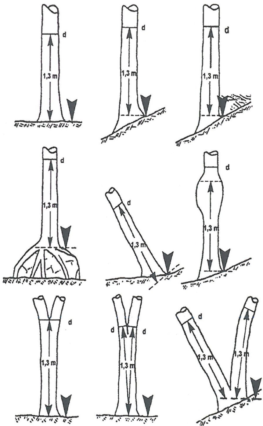
2. ábra Az átmérőmérés helyes végrehajtása
