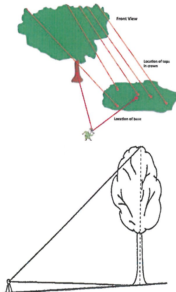
3. ábra A magasságmérés hibája a fa csúcsának meghatározásából eredően és a csúcs helyes meghatározása
