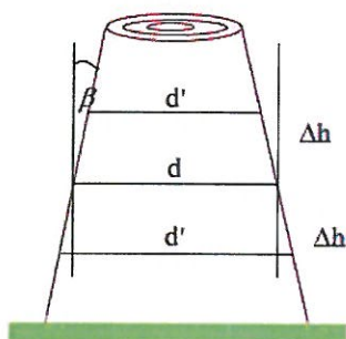
1. ábra A helytelen mérési magasságból eredő hiba
